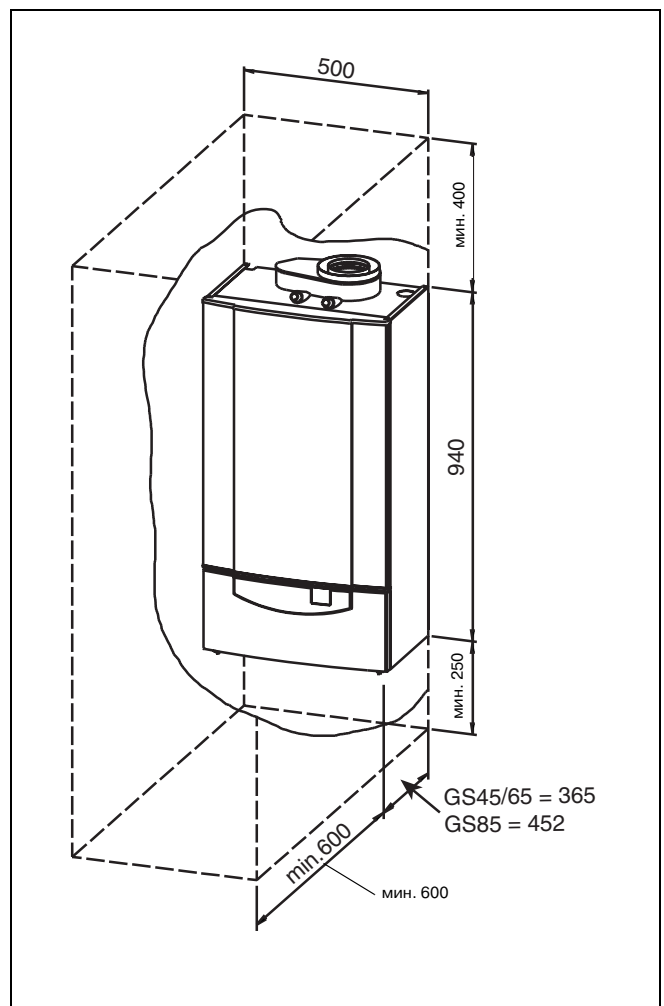
Илл. 6: Занимаемая котлом площадь при монтаже
