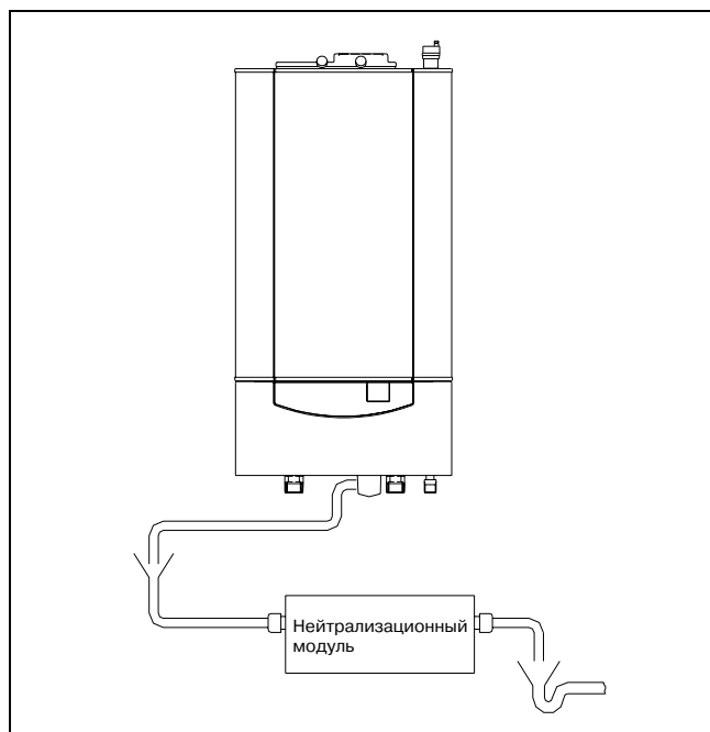
Илл. 7: Отвод конденсатных вод
