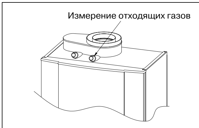
Илл. 17: Точка измерения отходящих газов
