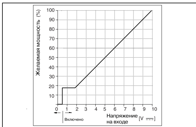
Илл. 13: Соотношение между напряжением на входе и мощностью котла
